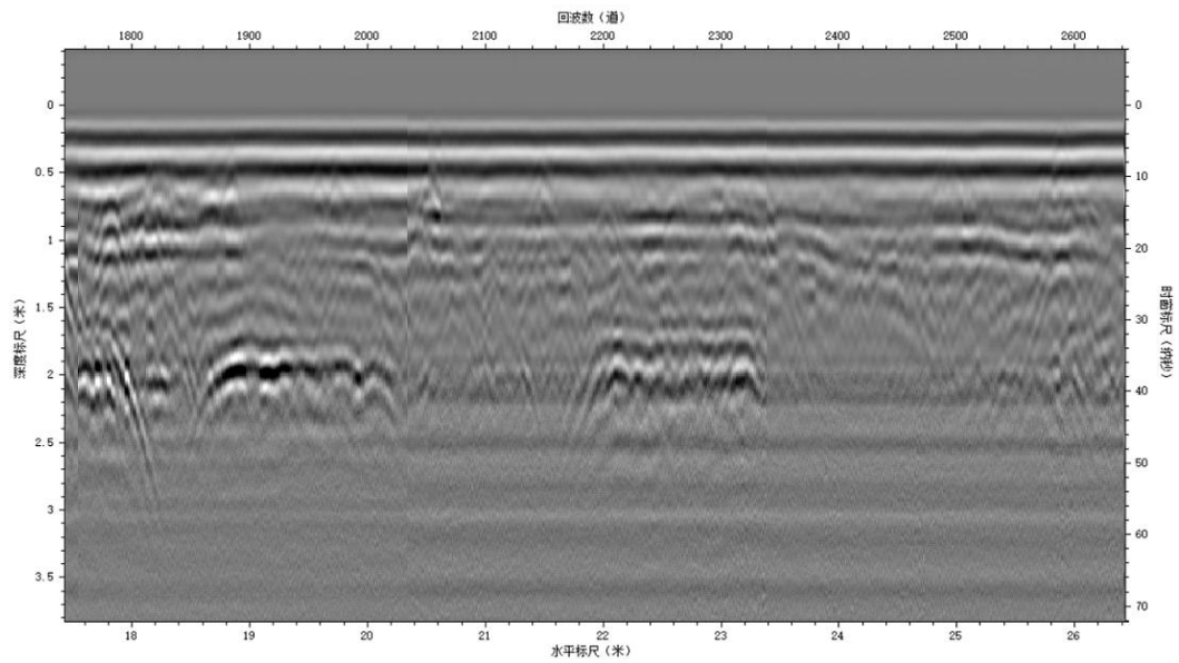
200MHz 雷达 道路暗涵测试
