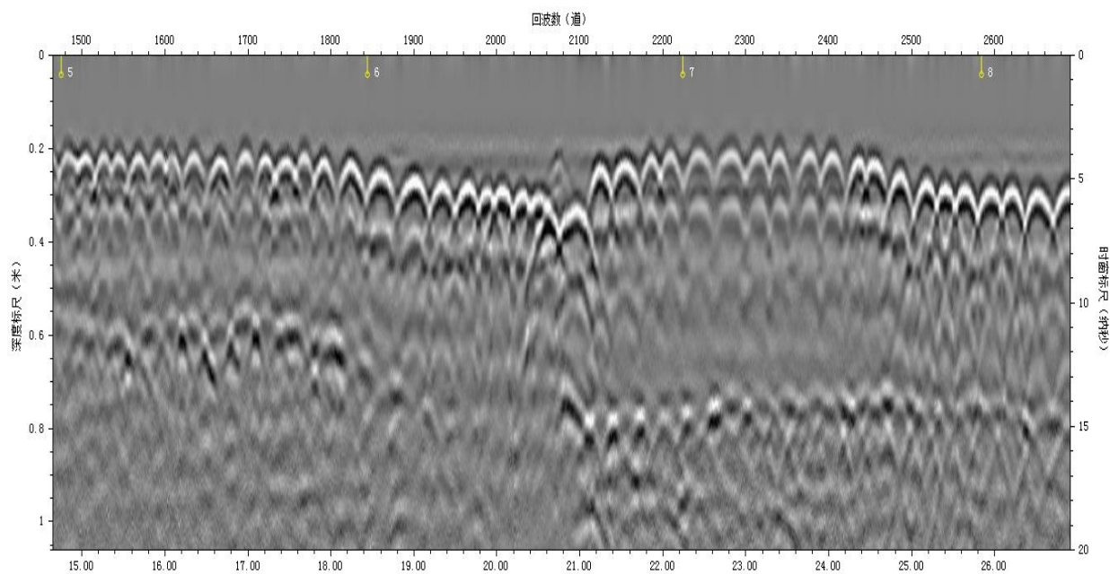
隧道衬砌检测数据
