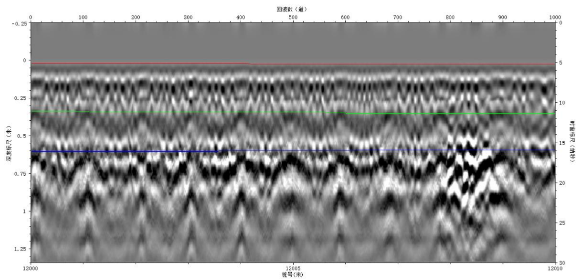
盾构隧道管片注浆检测效果
