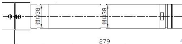
图3-2 ZKXG100-T尺寸
