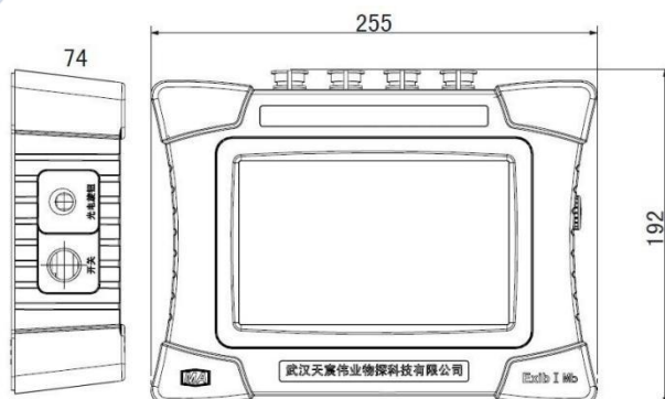
图3-1 主机尺寸
