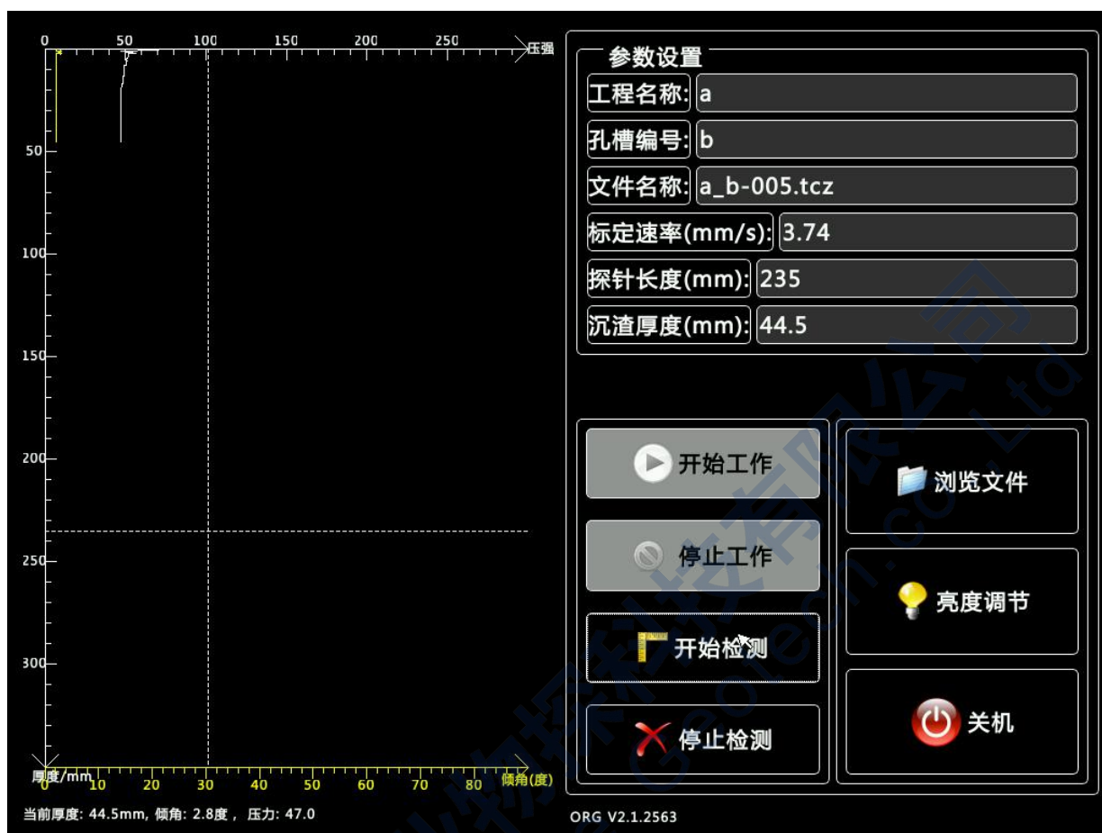
图3-19 沉渣采集界面
