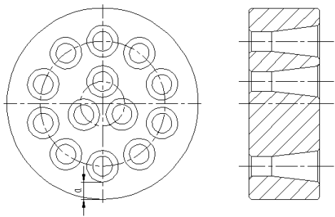
图1 锚板结构图
